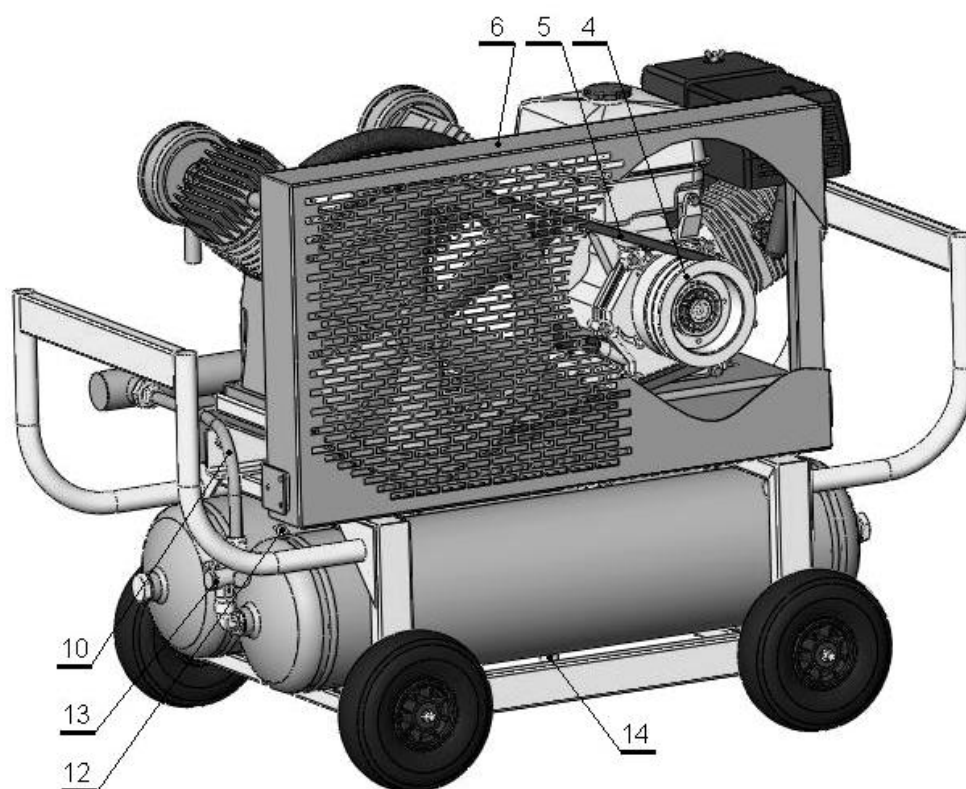
Рисунок 1 – Общий вид компрессорной установки
