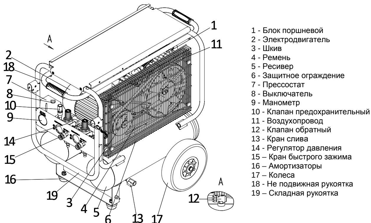
Рисунок 5 - Общий вид компрессора СБ4/С-23.LB30А
