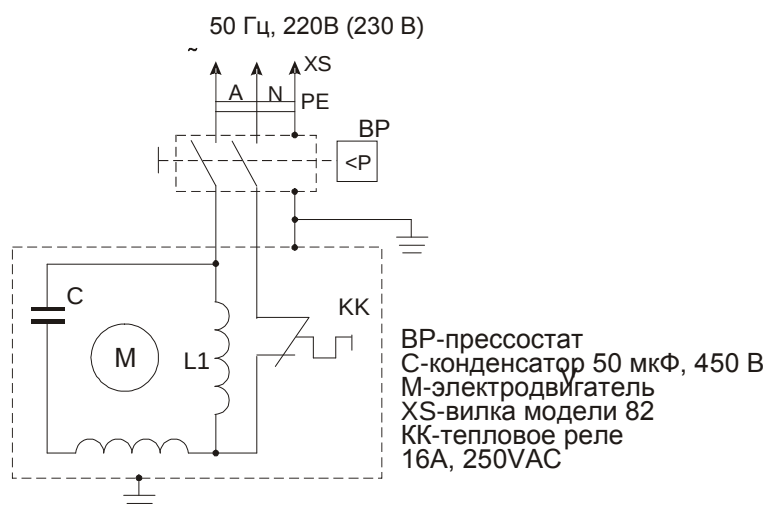
Рисунок А.1 - Схема электрическая принципиальная компрессора СБ4/С-23.LB30А
