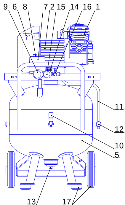
Рисунок 10 - Общий вид компрессора CB4/C-50.J2047BV
