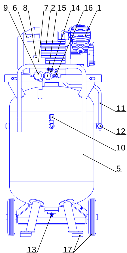
Рисунок 10 - Общий вид компрессора CB4/C-100.J2047BV
