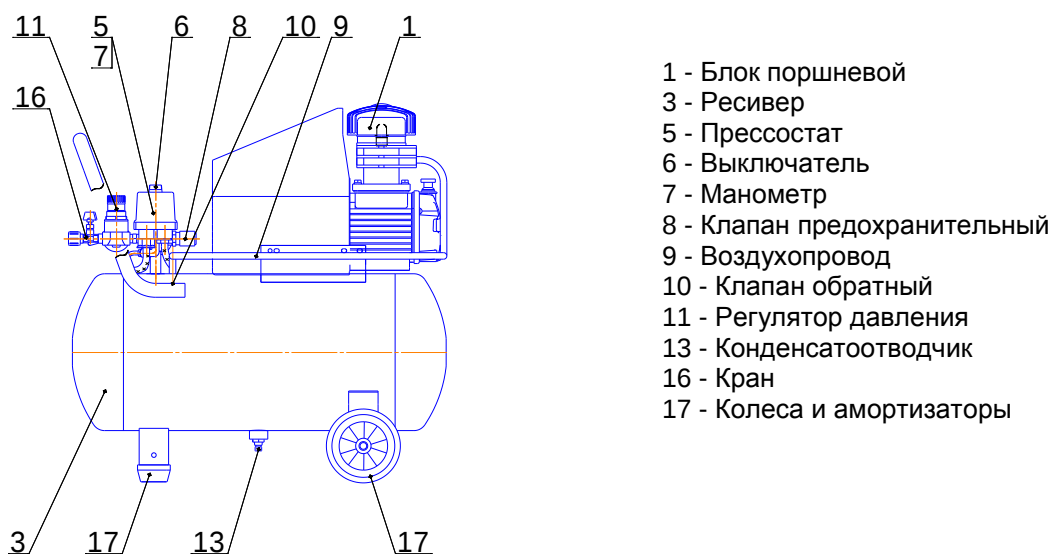
Рисунок 4 - Общий вид компрессора СБ4/С-24.J1047В
